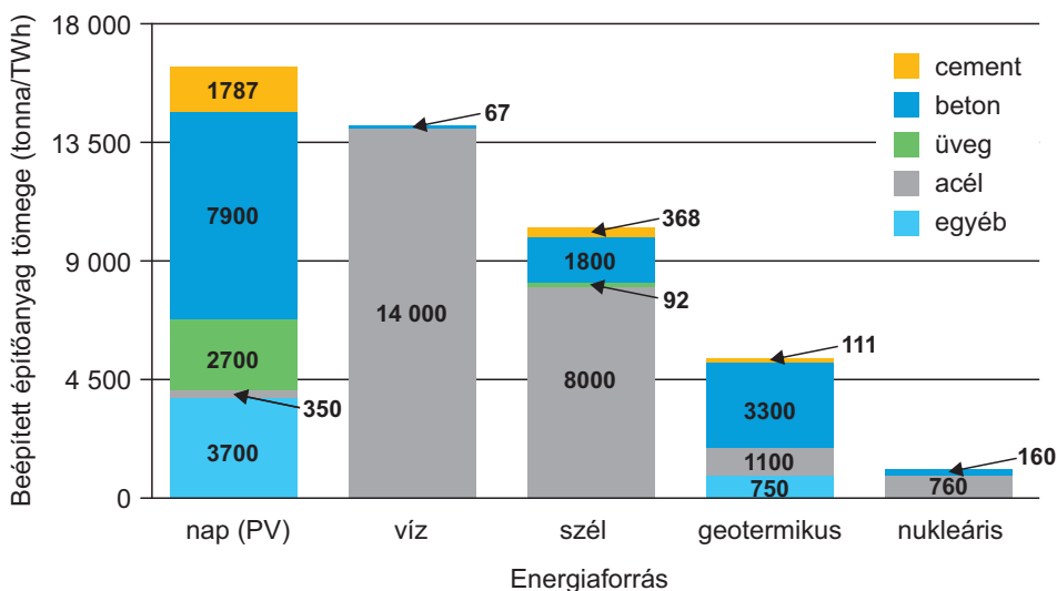
3. ábra. Az egyes energiaellátási megoldásokkal egy-egy TWh-nyi kapacitás létesítésénél fellépő fajlagos anyagszükséglet ábrázolása (DOE, 2015 nyomán).
