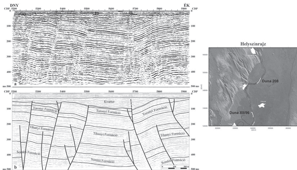
2. ábra. Korai többszornás vízi szeizmikus szelvény (Duna-208) a DH vető ÉK-i részén (Tóth, 2003 alapján, módosítva). Az értelmezés szerint a pannóniai rétegeket (Somlói, Tihanyi és Toronyi Formáció) markánsan elnyíró vetők érintik a pannon tetejét jelző diszkordanciafelületet, valamint a kvarter összlet alsó részét is
