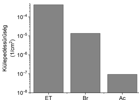
2. ábra. A belélegzett cseppek kiülepedéssűrűsége a felső légutakban (ET), valamint a tüdő bronchiális (Br) és acináris (Ac) régiójában. Fontos észrevenni, hogy itt az y tengely logaritmikus (a szerző szerkesztése)
