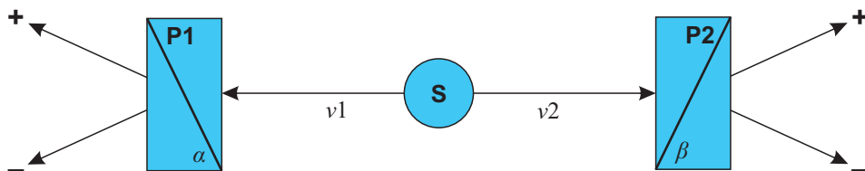
1. ábra. Alain Aspect kísérletének sémája
