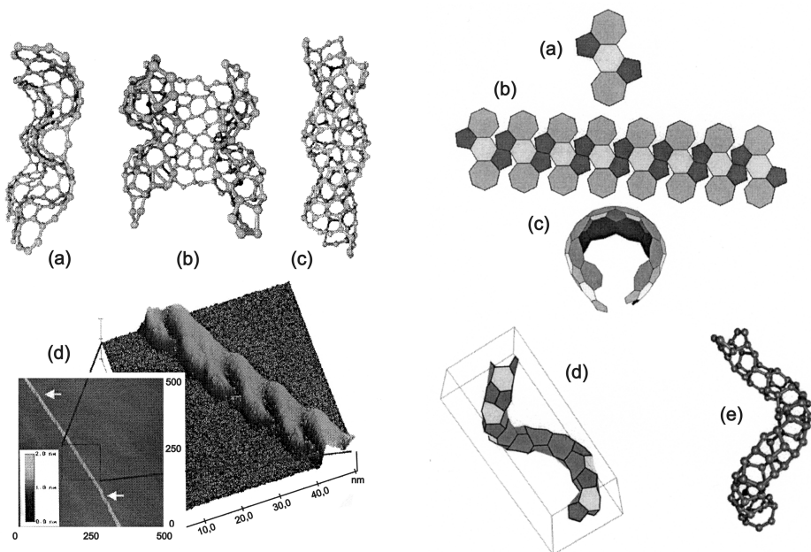
6. ábra • Haeckelite típusú egység, szalag és felület. a) Egy hatszöggel elválasztott két azule-noid elemből álló egység; b) az egység egyik lehetséges elrendezésével épített szalag; c) a b)-ben látható szalagot alkotó sokszögek éleinek összeillesztésével létrehozott görbült felület, a felület belső oldalát jelölő szürke árnyalatok sötétítettek; d) és e) a c)-ben ábrázolt felület csővé zárásával keletkező szabályos nanocső spirál kétféle ábrázolásban (Biró, 2002c) nyomán.
