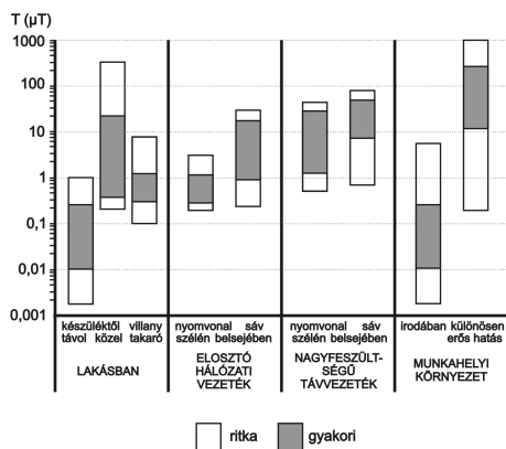
13. ábra • A hálózati frekvenciás mágneses erőter jellegzetes forrásai által létrehozott indukció összehasonlítása
