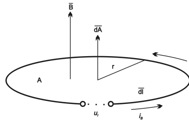
8. ábra • A mágneses erőter által indukált test-örvénnyáram kialakulásának mechanizmusa
