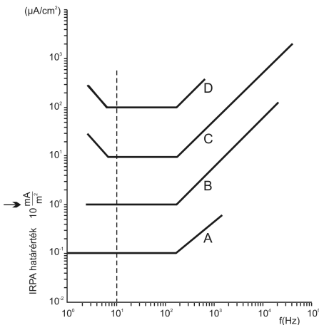
A – nincs biológiai hatás (a természetes agyáramsűrűség átlaga) B – jól meghatározott hatások, beleértve a látási és idegrendszeri hatásokat C – ingerlékeny szövet izgatása (a lehetséges egészségi kockázat határa) D – extra szívösszehúzódnás és szívkamrarelebegés (akut egészségi kockázat határa)
