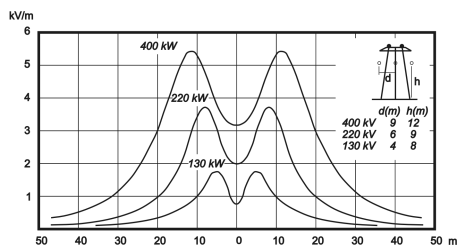
10. ábra • Különböző feszültségű távvezetékek jellemző villamos térerősség értékei a nyomvonalra merőleges irányban, 1,8 m magasságban
