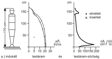
7. ábra • Villamos erőter hatására
