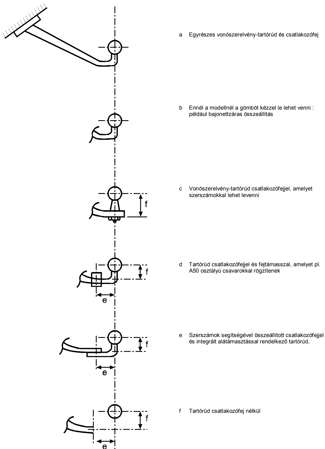
20. ábra – Csatlakozófejes vonószerelvénymű-tartó rudak kialakításai
