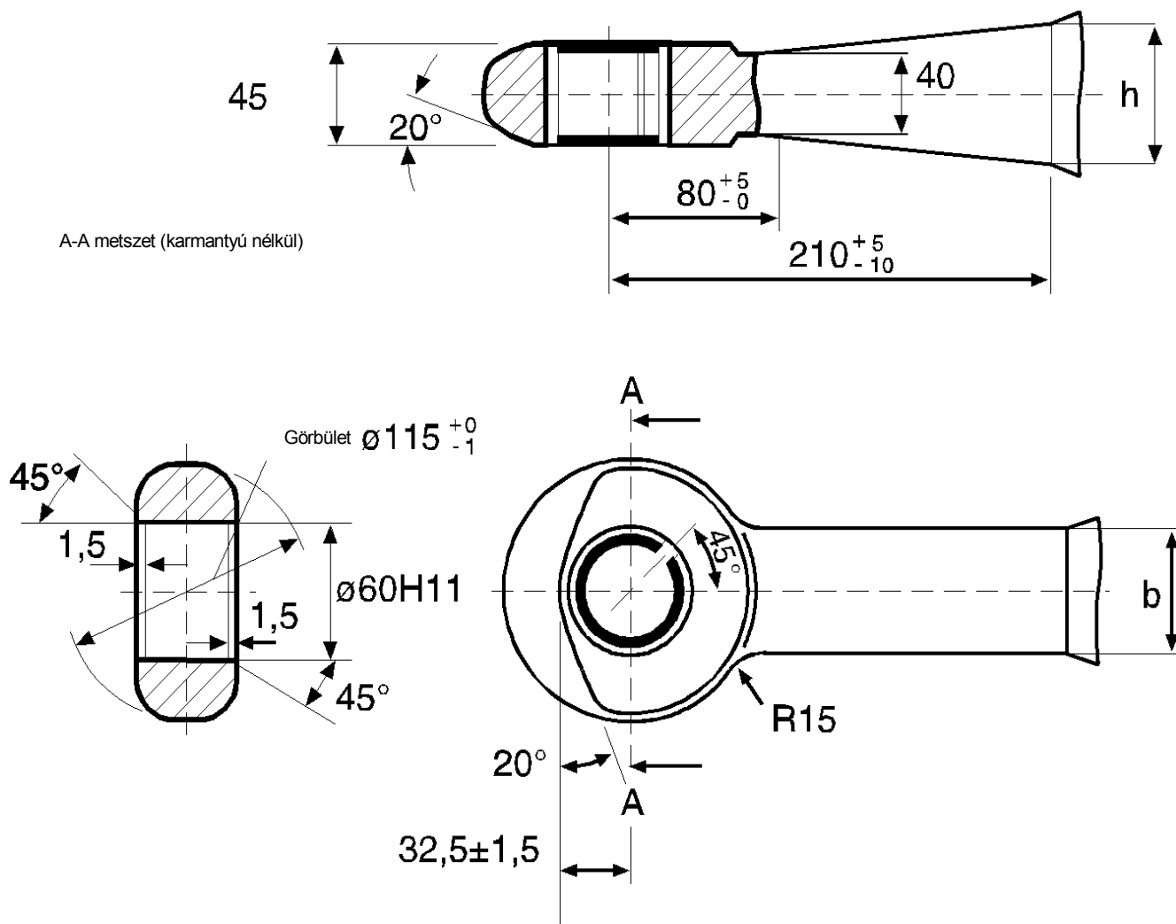
11. ábra – D50-A és D50-X osztályú vonórúdszemek méretei, lásd 6. táblázat
