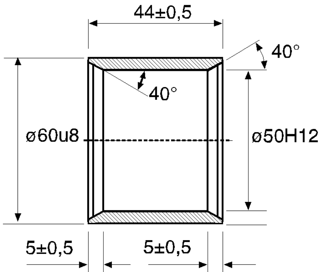
10. ábra – D50 osztályú vonórúdszemek nem hasított karmantyúja
