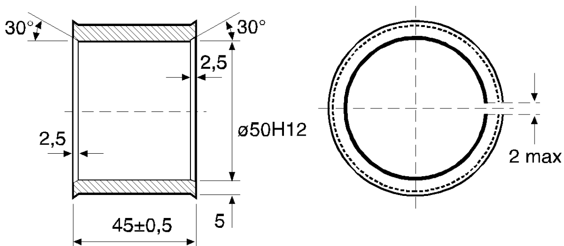
9. ábra – D50 osztályú vonórúdszemek hasított karmantyúja
