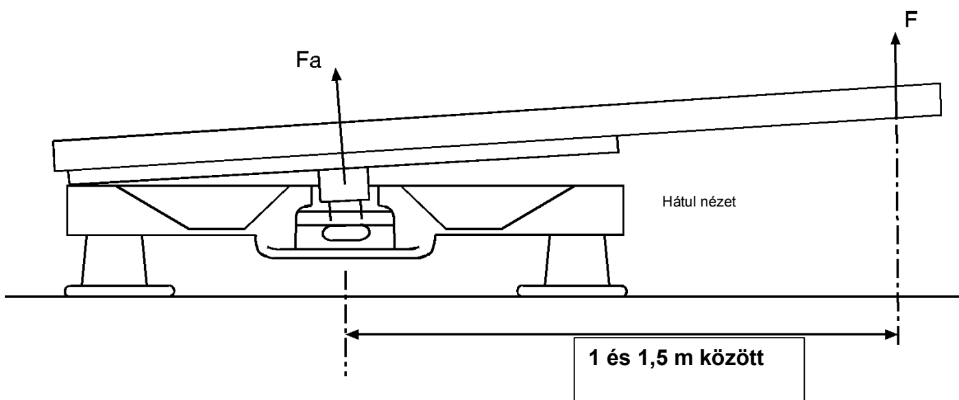
24. ábra – A nyerges vontató emelőtesztje
