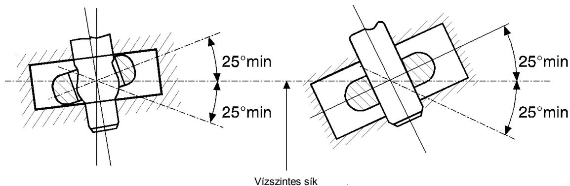
7. ábra – A csatlakoztatott vonórúdszem axiális forgása
