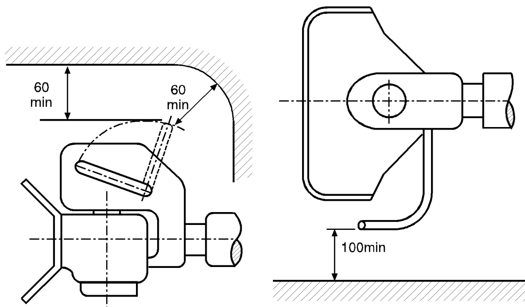
26. ábra – A kar körüli szabad tér
