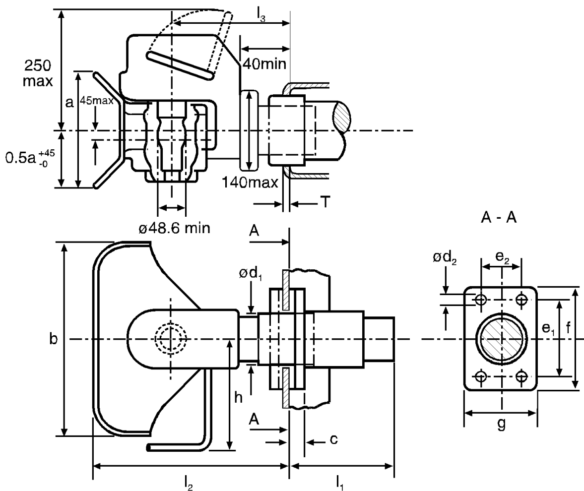
8. ábra – Szabványos vonórúd-csatlakozás méretei (mm), lásd 4. táblázat
