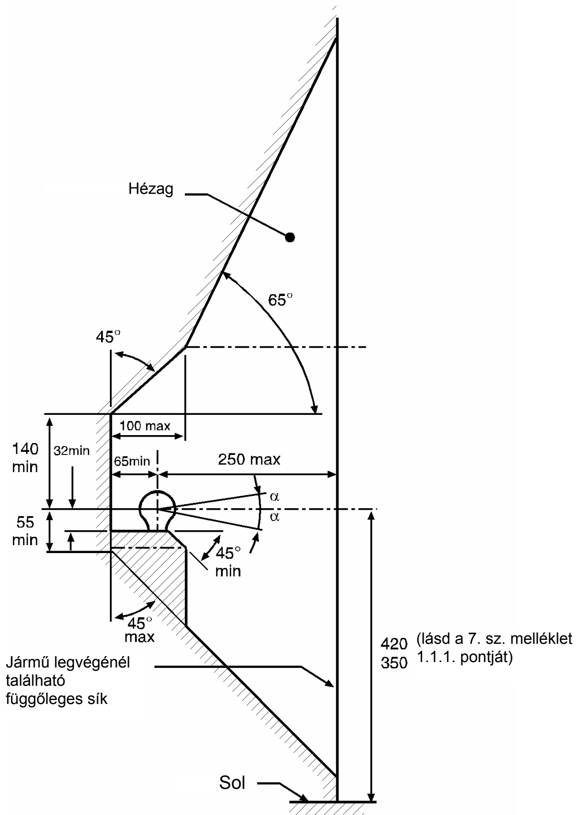
25. (a) ábra – A csatlakozófej hézaga és magassága – oldalnézet
