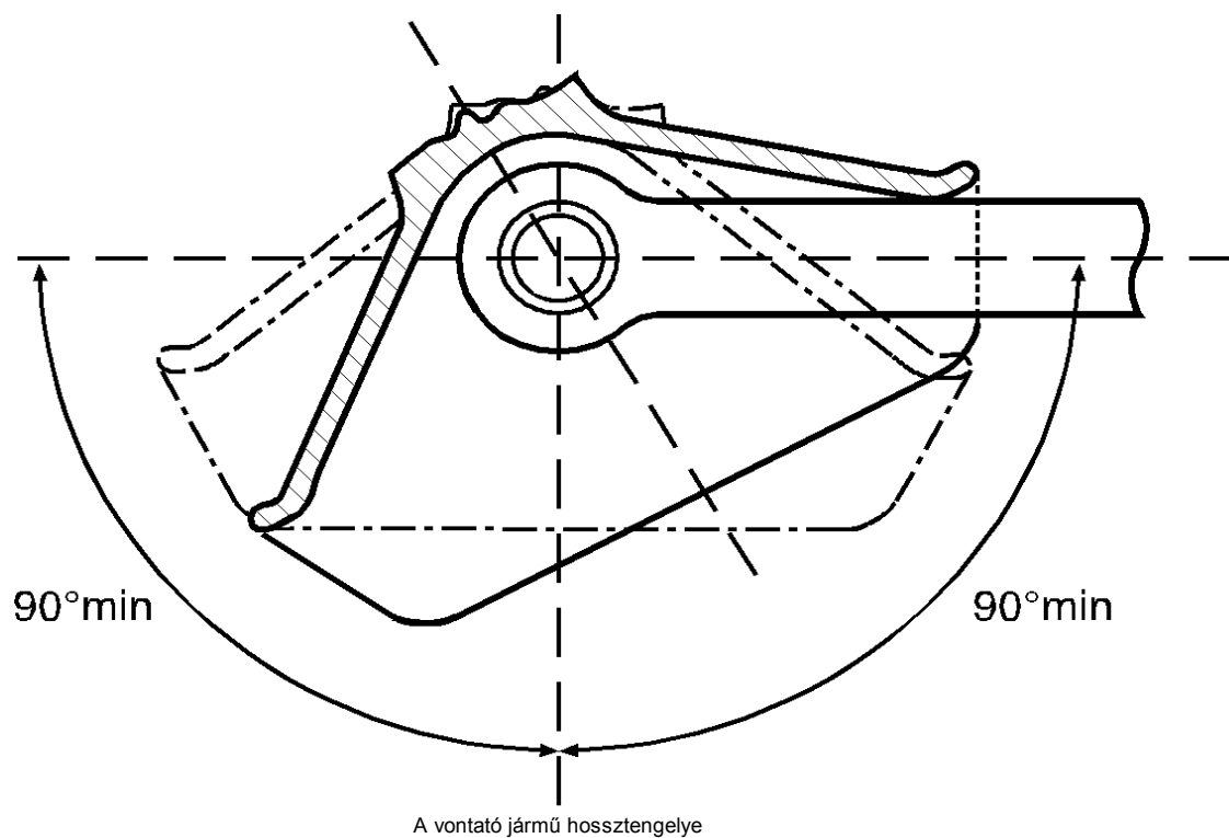
5. ábra – A csatlakoztatott vonórúdszem vízszintes forgása
