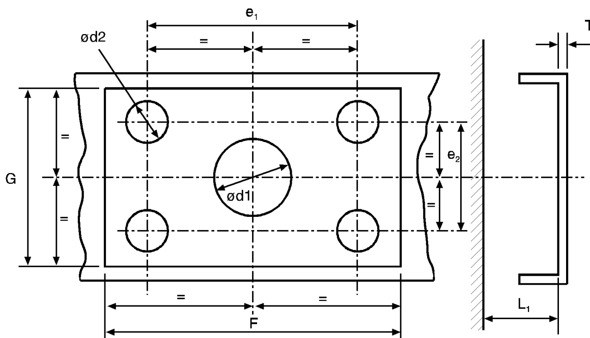
15. ábra – Szabványos vonórúd-csatlakozás szerelési méretei (lásd a 10. táblázat)
