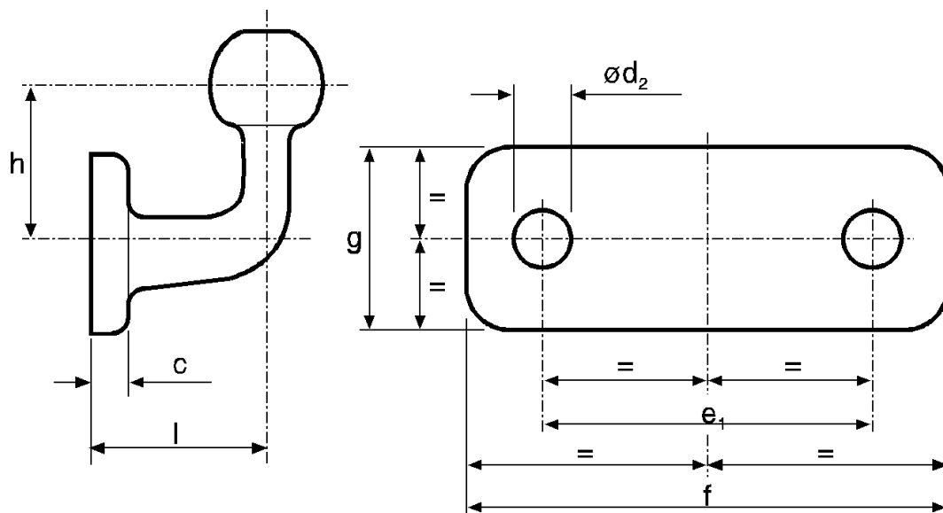
3. ábra – A A50-1 osztályú szabványos karimás csavarozott rögzítésű csatlakozófej méretei
