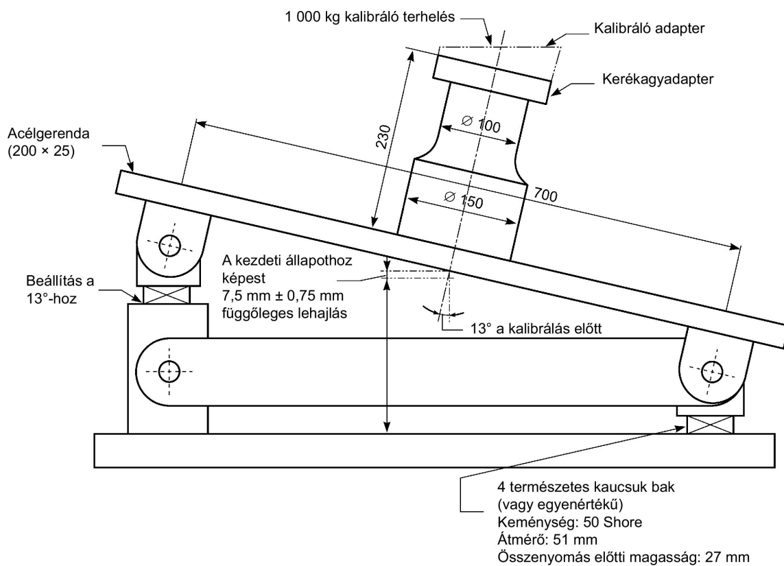
2. ábra: A terhelés működtetése a kerék tartóelemének közepén
