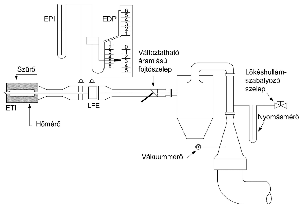
A CFV-CVS rendszer hitelesítésének konfigurációja
