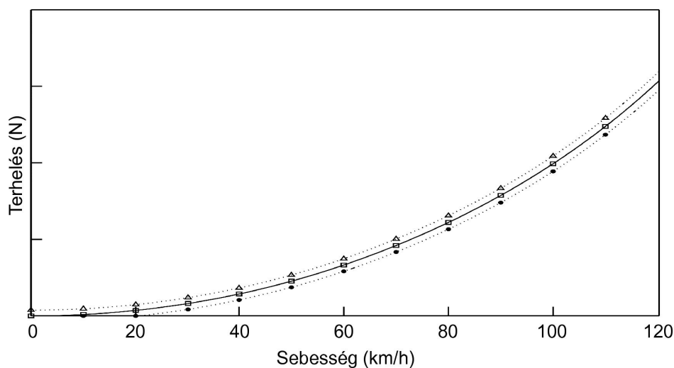
A görgős próbapad által elnyelt energiát szemléltető ábra
