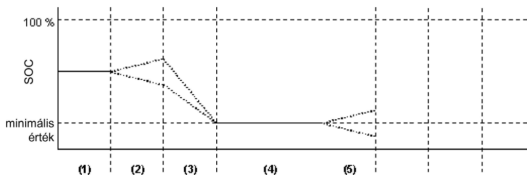
Az I. típusú vizsgálat B. feltétele
