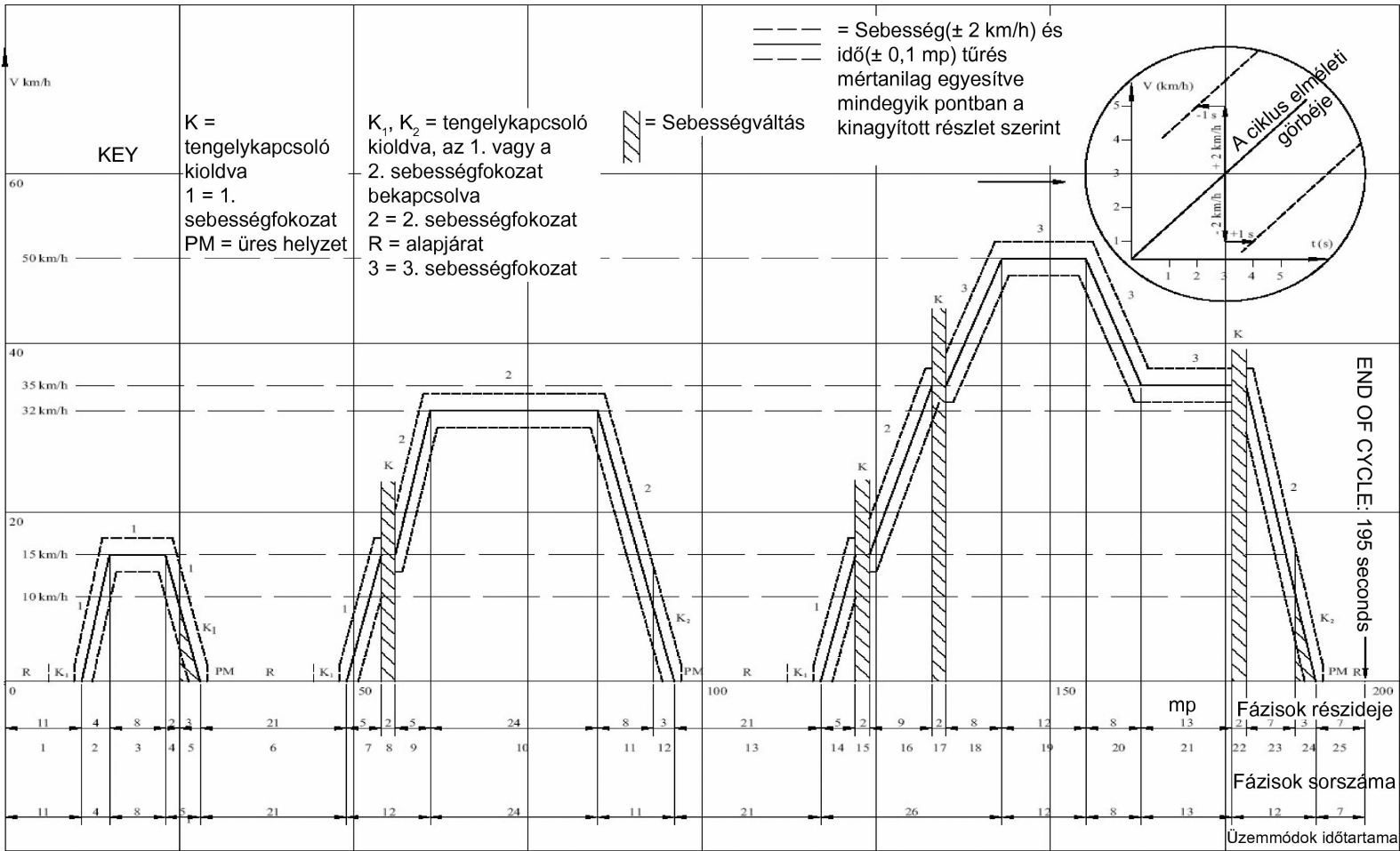
Az I. típusú vizsgálat alapvető városi ciklusa
