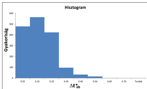
5. ábra. FD-9 spektrofotométer méréseinek hisztogramja
