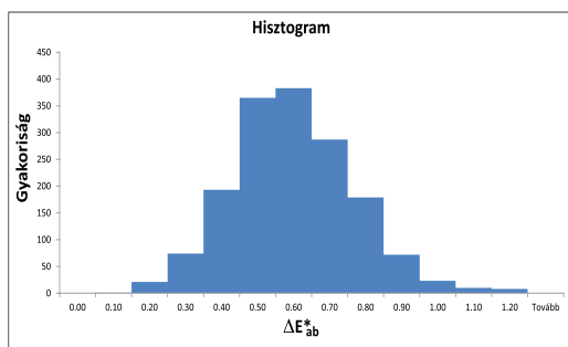
6. ábra. FD-7 spektrofotométer méréseinek hisztogramja
