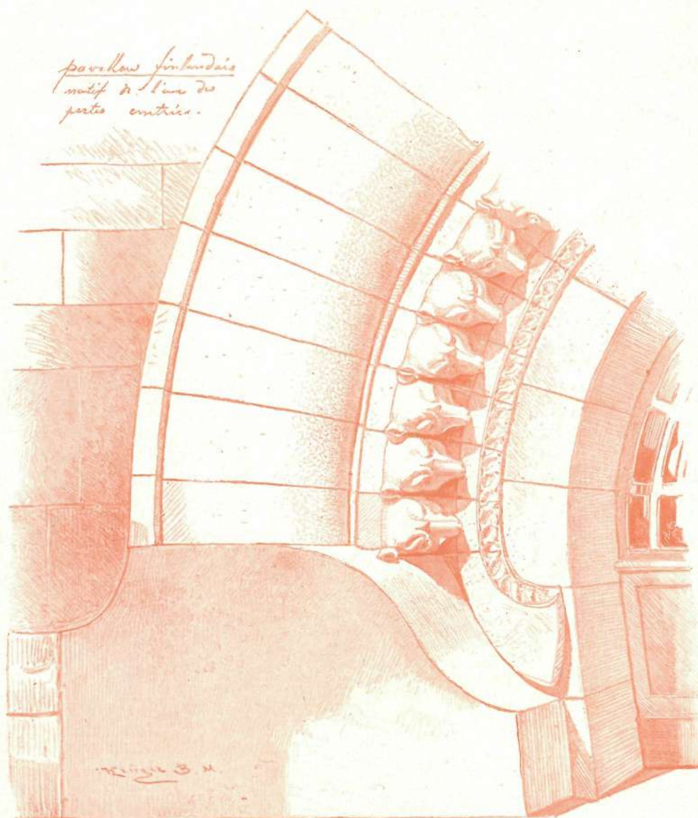
A FINN PAVILLON KAPUJÁNAK RÉSZLETE.
