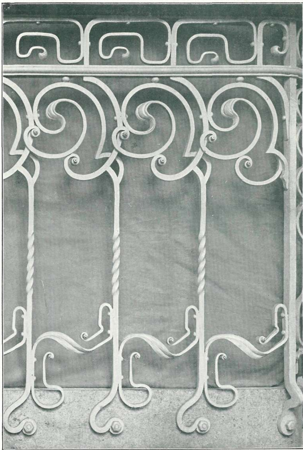
107. LÉPCSŐKORLÁT KOVÁCSOLT VASBÓL.
