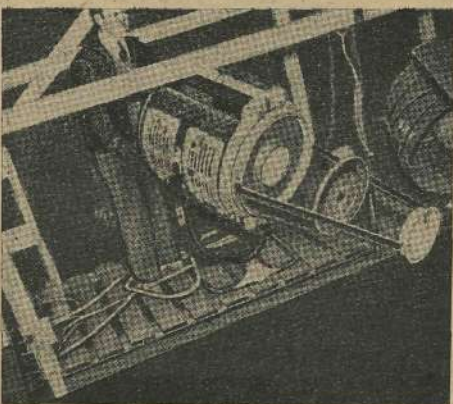
„Mole-Richardson 170” jelzésű hosszú gyűjtőtávolságú, különleges esetekben használt fényzó. Sugárkéveje hosszú távolságokra hat anélkül, hogy a kivetített fénymező éles határvonalait elveszítené.
