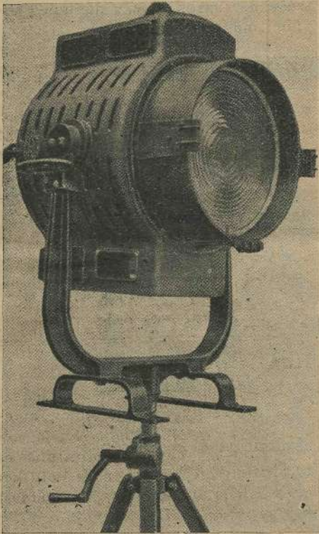
A müncheni Arnolt és Richter cég által gyártott 5000 W teljesítményű körbordás lencsés fényzó. Egyöntetű irányított fénye és a lámpaház tömör kivitele a korszerű jelenetbevilágítás minden követelményének megfelel.
