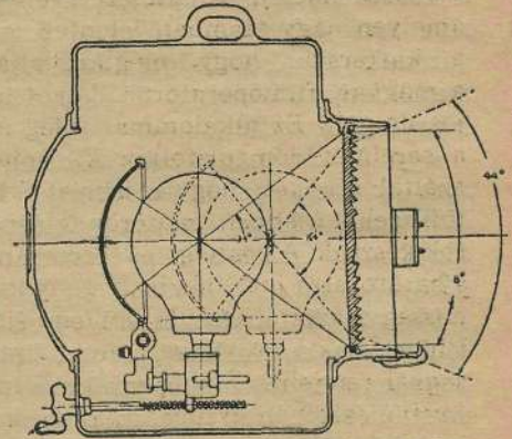
A tükrös, izzólámpa és a körbordás (Fresnel) lencse helyzete és a fényvisszaverődés szöge szórás és szűkítés esetében.
