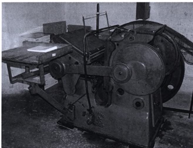
Tégelysajtó
