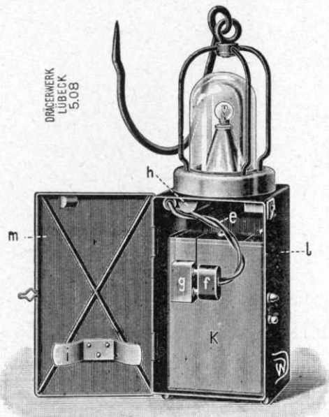
4. sz. rajz. Az új Dräger-lámpa, beállított akkumulátorral.
