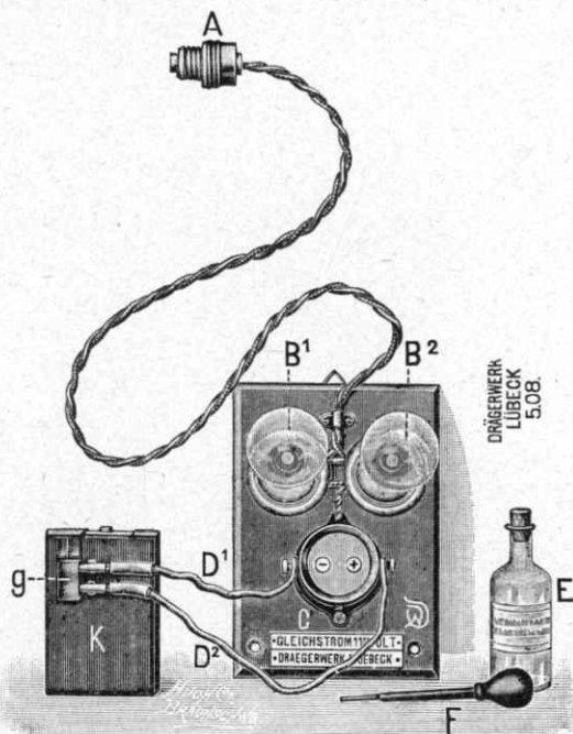
5. sz. rajz. Töltőkészülék a Dräger-lámpa-akkumulátorok számára.
