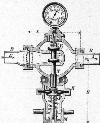
Dreyer, Rosenkranz és Droop-féle szab. víz- és levegő-nyomást csökkentő szelep.
