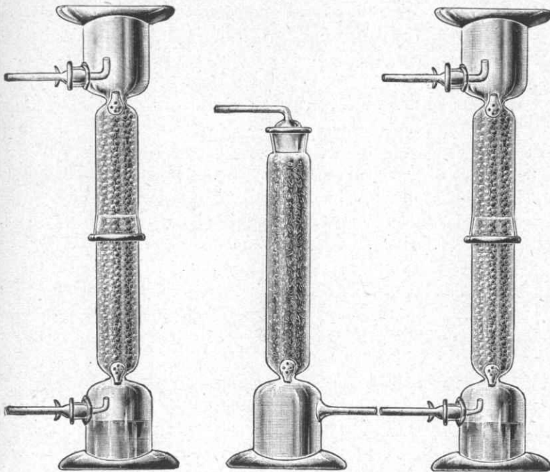
1. és 2. sz. rajz. Megfordítható kénsavtornyok.
