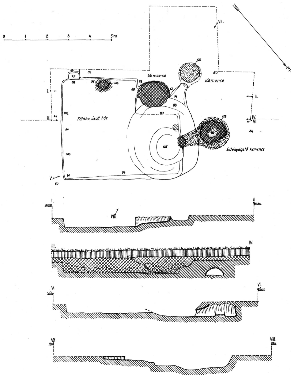
6. kép. Földbe ástott, szarmata kori lakóház és edényégető kémence alaprajza és metszetei. Hajdúirtás.
