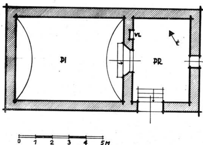
155. kép. Az előző képen bemutatott prэшáz alaprajza Abb. 155. Grundriss des Kelterhauses Abb. 154.
