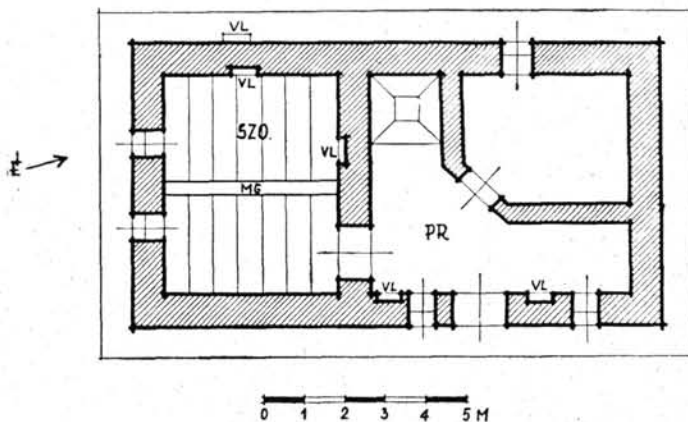
169. kép. Az előző prэшáz alaprajza
