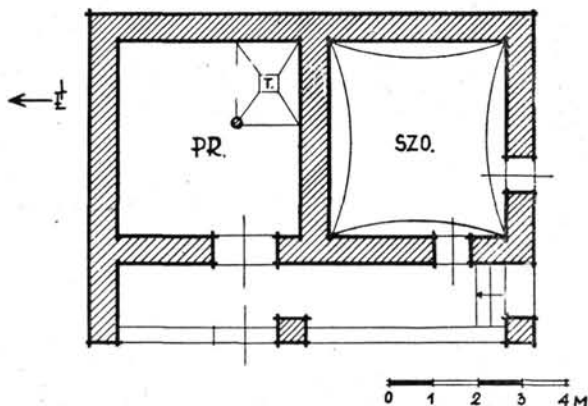
174. kép. Az előző prэшház alaprajza
