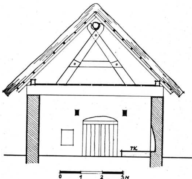
164. kép. Az előző préház tetőszerkezeti rajza Abb. 164. Dachkonstruktion des Kelterhauses Abb. 159.
