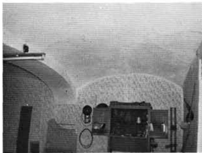
10. ábra. Csehüvegboltozatú födém Borbély Gyula köveskál házában
