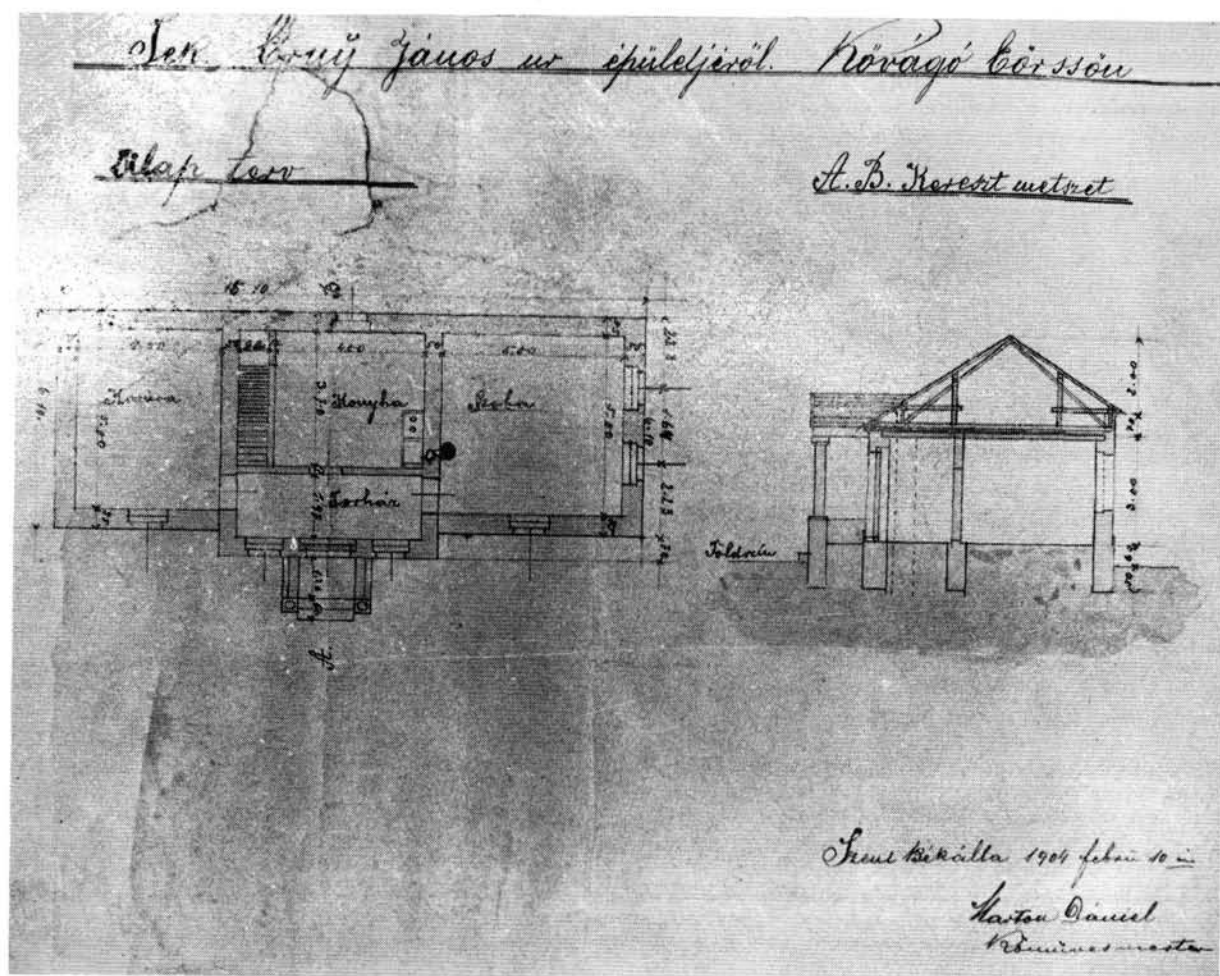
26. ábra. Marton Dániel kőművesmester tervrajza 1904-ből Erny János kővágóörsi házáról Abb. 26. Bauplan des Maurermeisters Dániel Marton vom Jahre 1904 über das Haus von János Erny in Kővágóörs.
