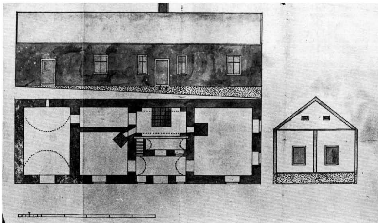
25. ábra. Marton Dániel szentbékai kőművesmester tervrajza kétszobás, szabad kéményes konyhájú, dongaboltozatos kamrájú házról
