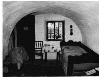
10. ábra. Csehüvegboltozatú födém Borbély Gyula köveskál házában
