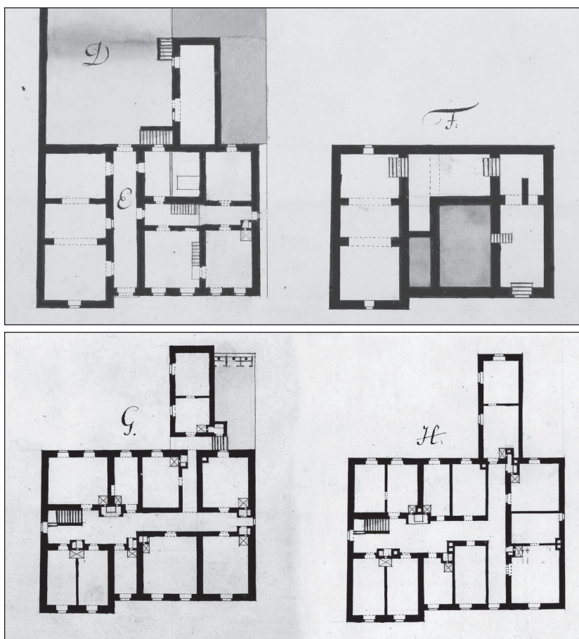
1/a ábra: A Kolleum alaprajza (1773 után, részletek)
