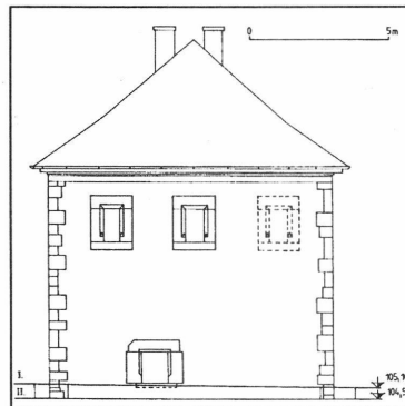
3. kép. Az 1500 után épült ház északi fala. Nézeti rajz
