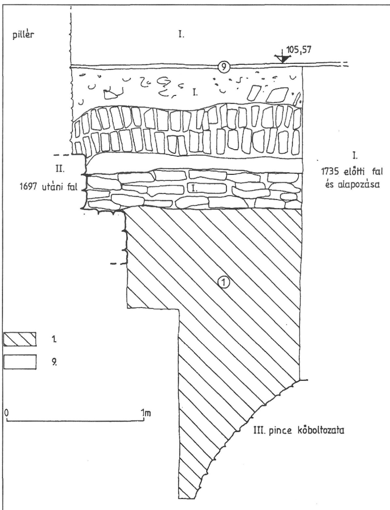
20. kép. Kelet-nyugati irányú metszet a pinceboltozattal, a 2. helyiségben. Rétegek I., 9. beton
