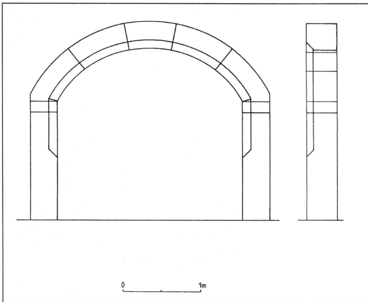
11. kép. A középkori kapu felmérési rajza
