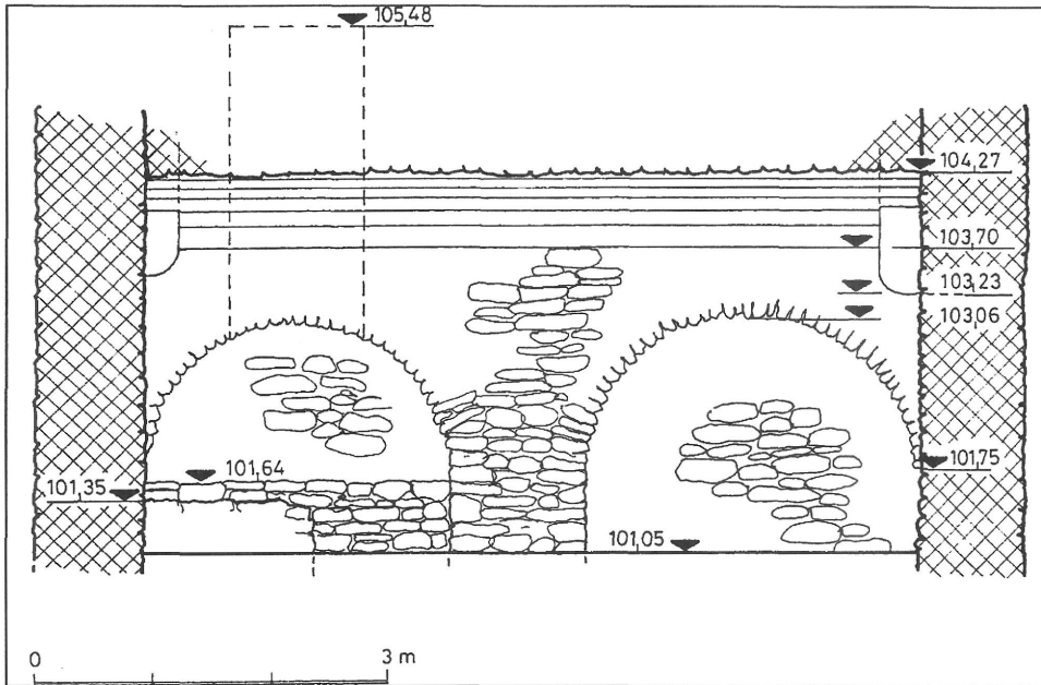
25. kép. A pince hosszmetszete
