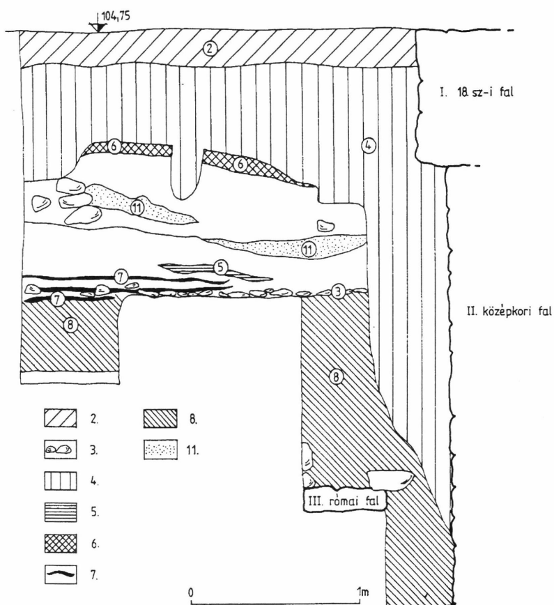
16. kép. Észak-déli metszet a Zichy u-i szárny déli falával. Rétegek: 2. törmelékenes barna föld. 3. kövek (út réteg). 4. kevert agyagos. 5. sárga agyag. 6. vörösrre átégett agyag. 7. korom sáv. 8. sötétbarna agyagos. 11. sűrű habarcsos (építési réteg)
