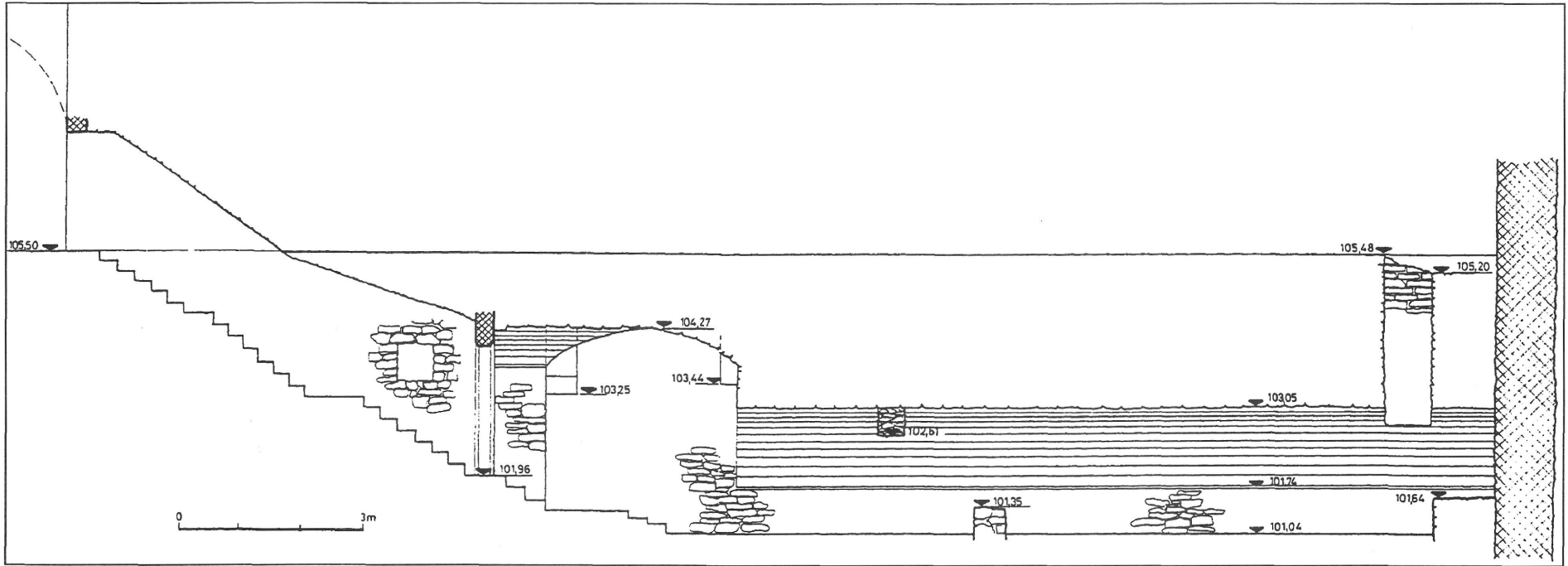
25. kép. A pince hosszmetszete
