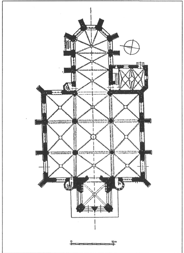
2/b. kép. A nürnbergi Frauenkirche alaprajza (Bräutigam 1965 nyomán)
