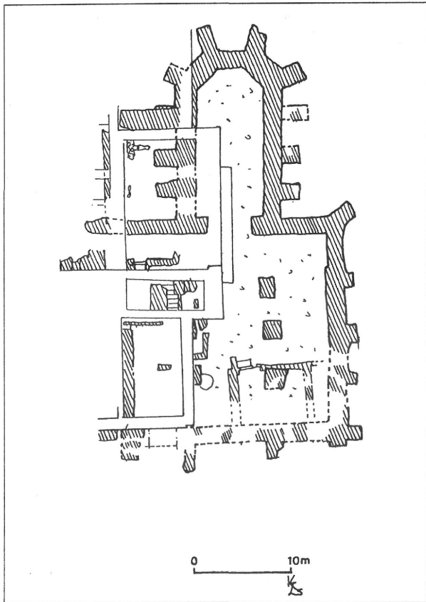
2/a. kép. A kisebb Szűz Mária (Szt. Zsigmond) templom alaprajza (Buzás–Feld 1996 nyomán)
