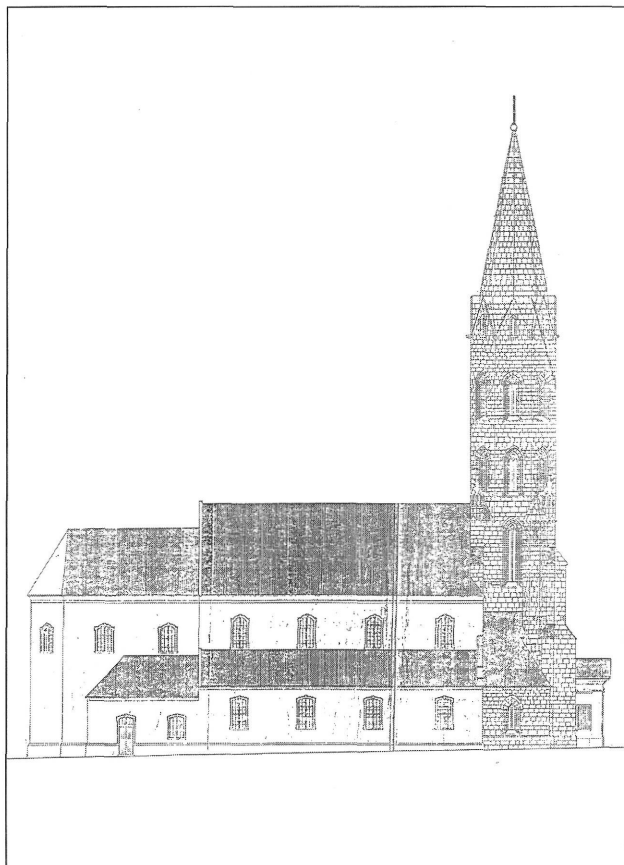
20. kép. Lux Kálmán jóváhagyott terve a Helyőrségi templom helyreállítására, északi homlokzat, 1946.
