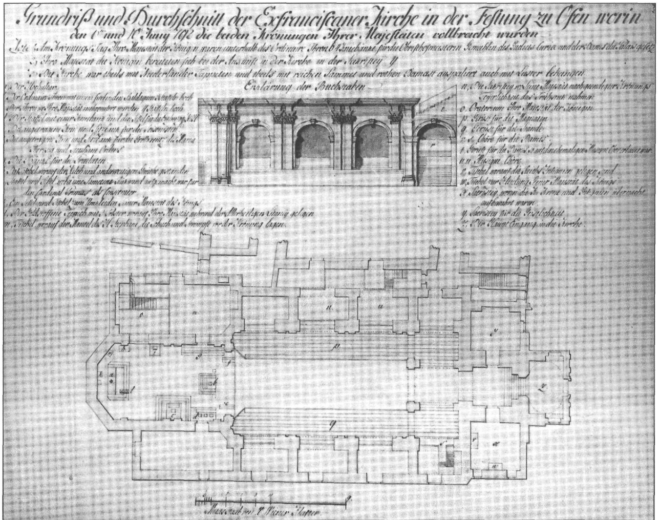
8. kép. A volt ferences templom alaprajza és a hajó metszete I. Ferenc koronázásakor, 1792-ben.
