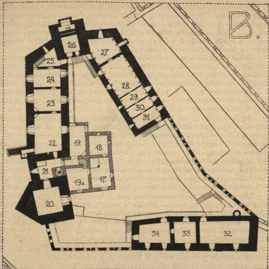
A VISEGRÁDI FELLEGVÁR I. EMELETI ALAPRAJZA A XV. SZÁZAD DEREKÁN.
