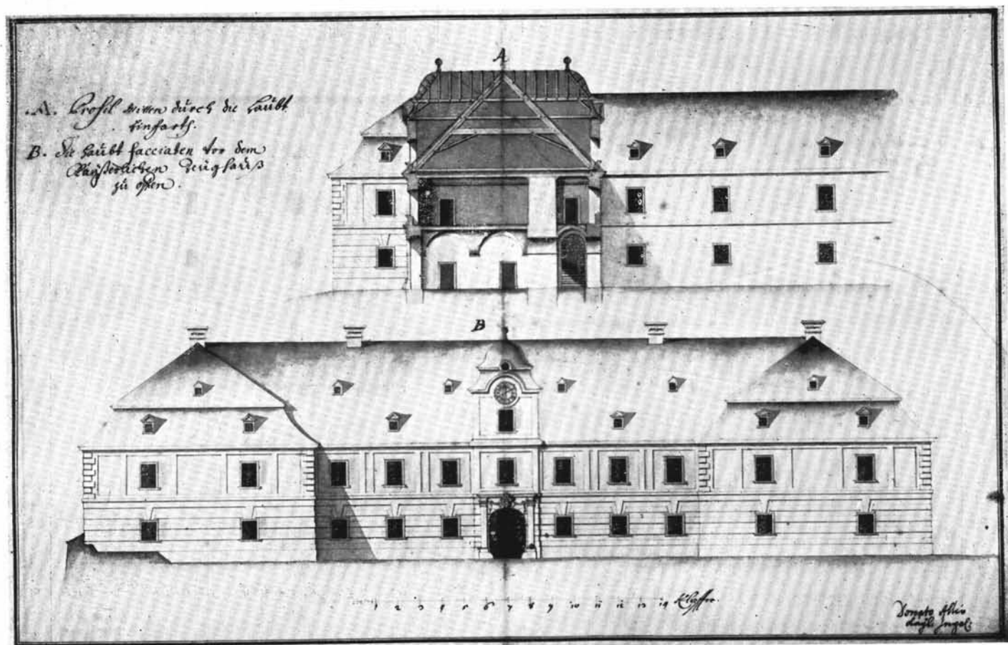
35. Allio főhomlokzat terve (8. tervrajz).
