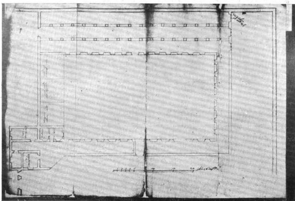
31. A budavári katonai szertár belső homlokzata és alaprajza a XVII. század végén
