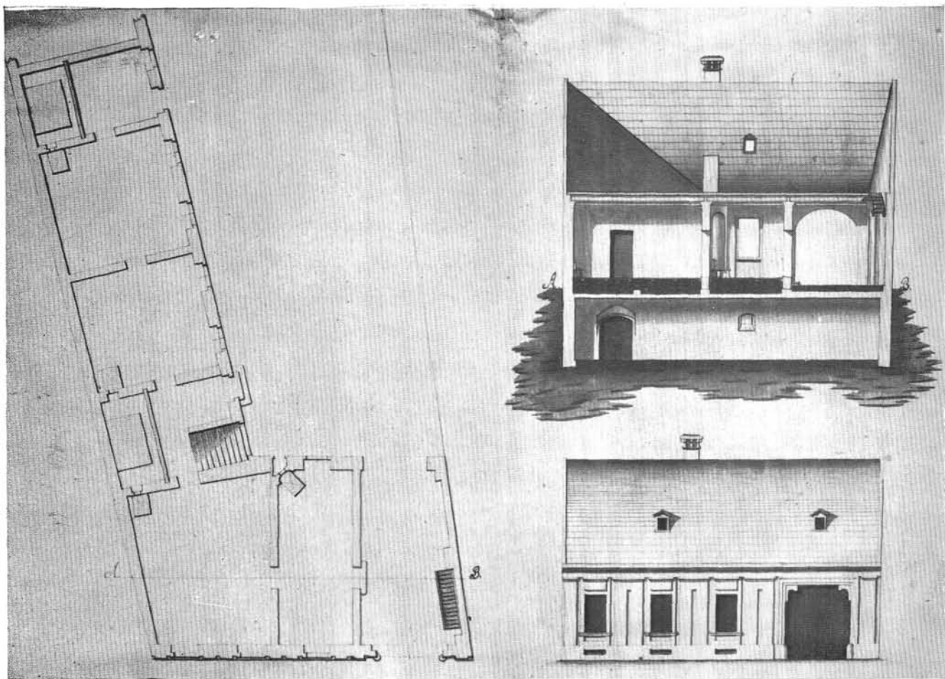
16. kép. II. Mártírok útja 14. Id. Eckermann József terve
