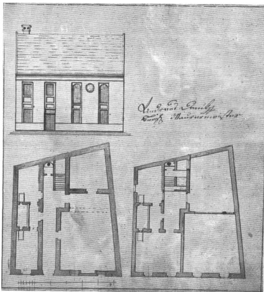
12. kép. I. Öntőház u. 5—7. Dankó András terve
