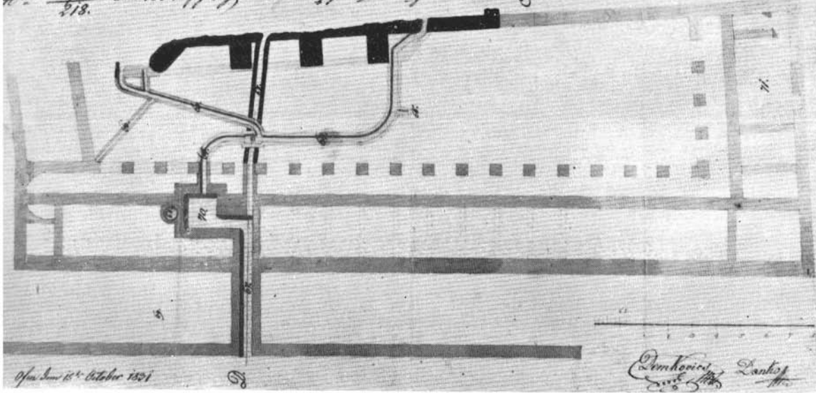
23. kép I. Döbrentei tér 9. Rudas-fürdő. Ifj. Dankó József terve
