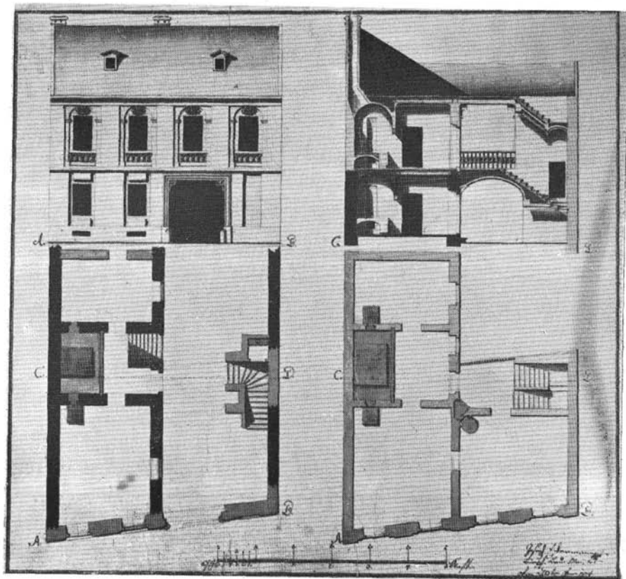
13. kép. II. Csalogány u. 13. Id. Eckermann József terve
