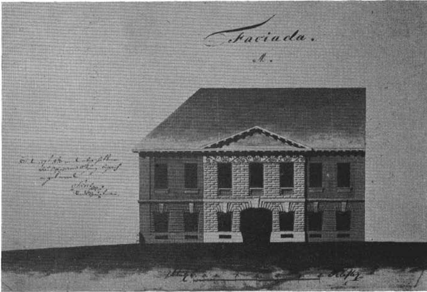
1. kép. I. Országház u. 19. Homlokzat. Eberl Carlo terve
