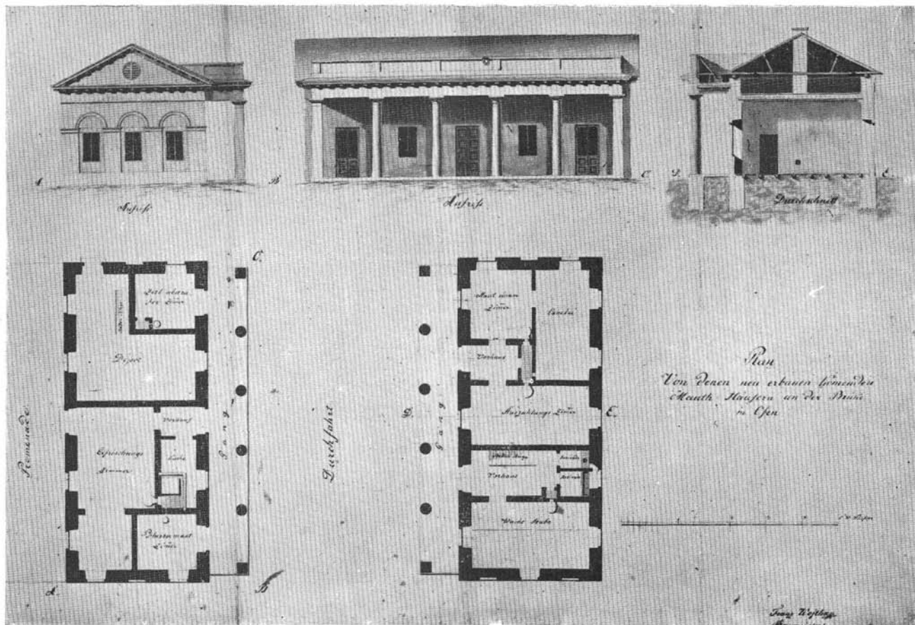
24. kép. I. Hajóhid őrháza. Wjthya Ferenc terve
