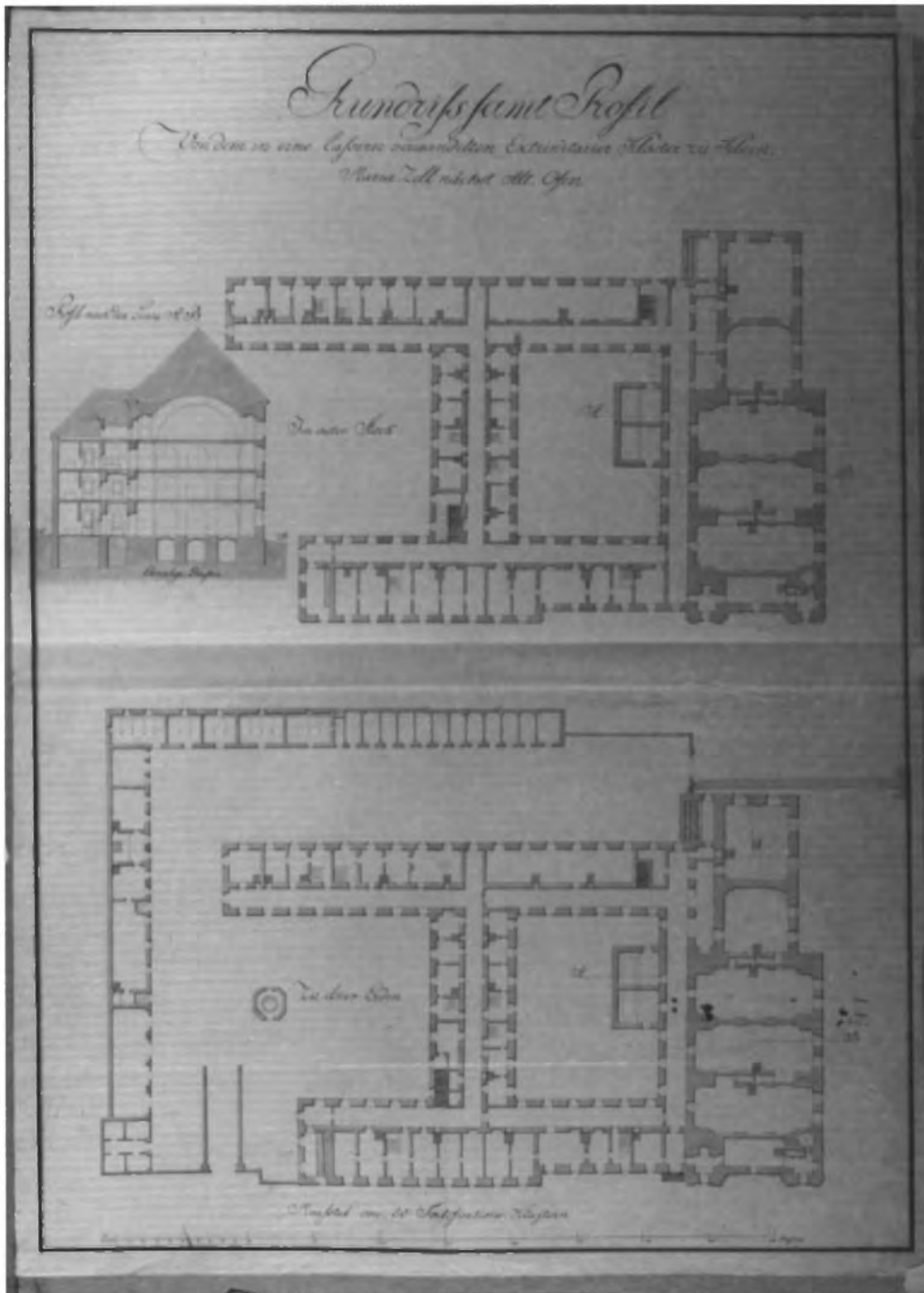
A kiscelli kaszárnya felmérési rajza, a földszinti és az emeleti alaprajzok, 1806? Készítette: Anton Gillet (Österreichisches Staatsarchiv, Kriegsarchiv, Kartensammlung, GVII, 1806-D-150)
