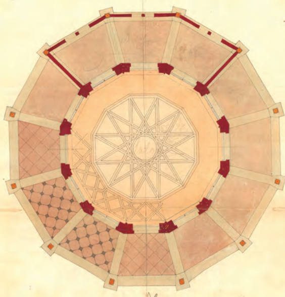
5. A kioszk összképe és a mennyezet nézete. Feszl Frigyes, 1860. BFL XV.17.b.314 77/e
