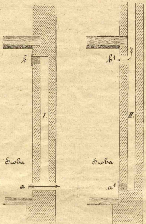
2. ábra. A szellőző működése nyáron.
