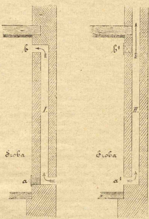
3. ábra. A szellőző működése télen.
