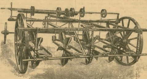
52. ábra. A Laass-féle burgonyalyukgató gép.
