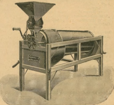
128. ábra. Kühne E. féle PN jegyű egyszerű működésű trieur (Konkolyozó.)
