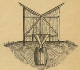
181. ábra. Kettősárnyékszék a trágyalé kutra.
