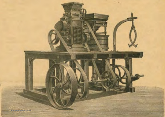
163. ábra. Ganz-féle kombinált szállítható malom hengerszek és kérel.
