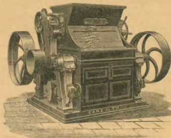
159. ábra. Ganz-féle kéthengeri darálószék.
