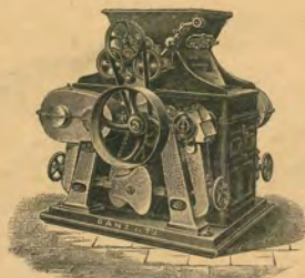
158. ábra. Ganz-féle négyhengeri vízszintes darálógöngyök.
