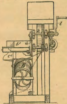
299. Ábra. Konkolyválasztóval kombinált gabonaszitógép. (Látó keret.)
