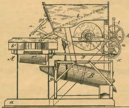
298. Ábra. Konkolyválasztóval kombinált gabonaszitógép. (Oldalnézet.)
