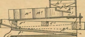
212. ábra. Konkolyválasztóval kombinált gabonatisztítógép. (Mészec a szitaszékrennyel át.)
