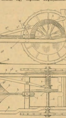
1. ábra. A Nick-féle burgonyakiszédgép oldalnézetben és felülnézetben.
