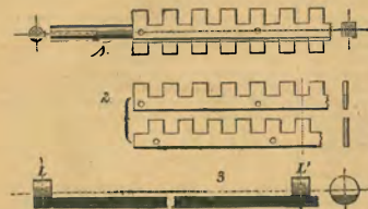
23. ábra. Schmitt és Spiegel-féle műtrágyaszórógép szóró- és zárótengelye.
