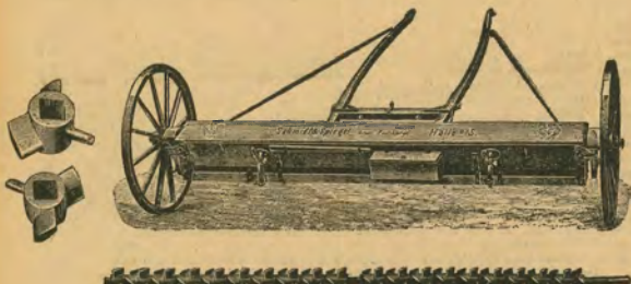
26. ábra. Schmitt és Spiegel-féle műtrágyaszórógép és keverőtengelye.
