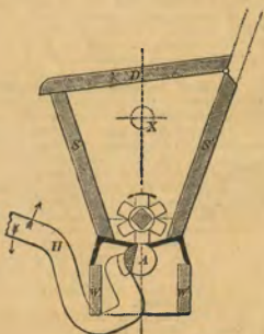
25. ábra. Schmitt és Spiegel-féle műtrágyaszórógép keresztmetszete.
