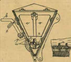
20. ábra. Dehne-féle műtrágyaszóró-gép vetőszekrénynek keresztmetszete.
