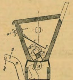
22. ábra. Schmidt és Spiegel-féle műtrágyaszóró-gép vetőszekrénynek keresztmetszete.
