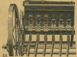
102. ábra. Sack IV. sz. toló kerekes hegyi vetőgépe hátdő részeknek bal felé.
