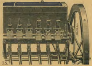
96. ábra. Sack IV. sz. toló kerekes hegyi vetőgépe hátdő részeknek jobb felé.
