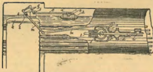
245. ábra. Önműködő vizszabályozó hosszmetézetben.
