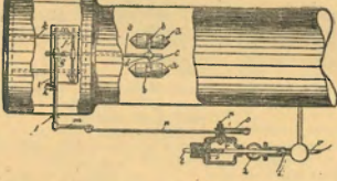
244. ábra. Önműködő vizszabályozó felülnezetben.
