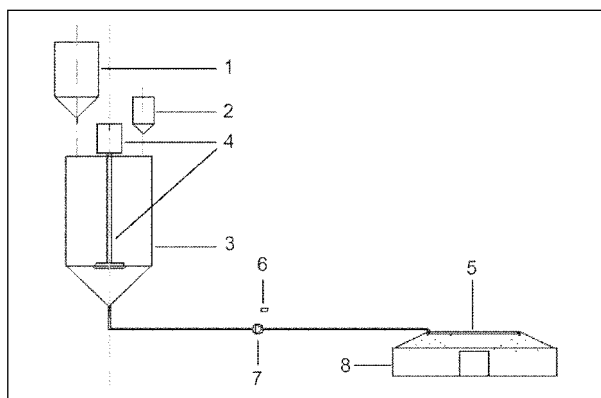
1. ábra. A pormegkötő berendezés elvi vázlata
