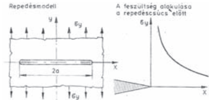
1. ábra Repedésmodell és feszültségkoncentráció Griffith szerint [8] Fig. 1. Crack modell and stress concentration according to Griffith [8]
