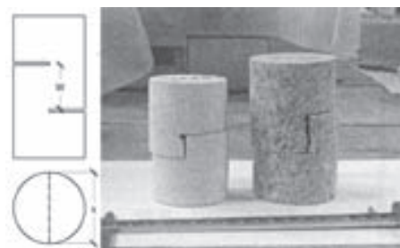
11. ábra Nyíróvizsgálat építőköveken [20] Fig. 11. Shear tests on structural stone specimens [20]
