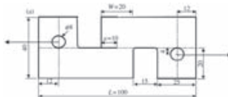
8. ábra Húzott polimer próbatest, K_{IC} meghatározásához [17] Fig. 8. Pulled polymer specimen for testing K_{IC} [17]
