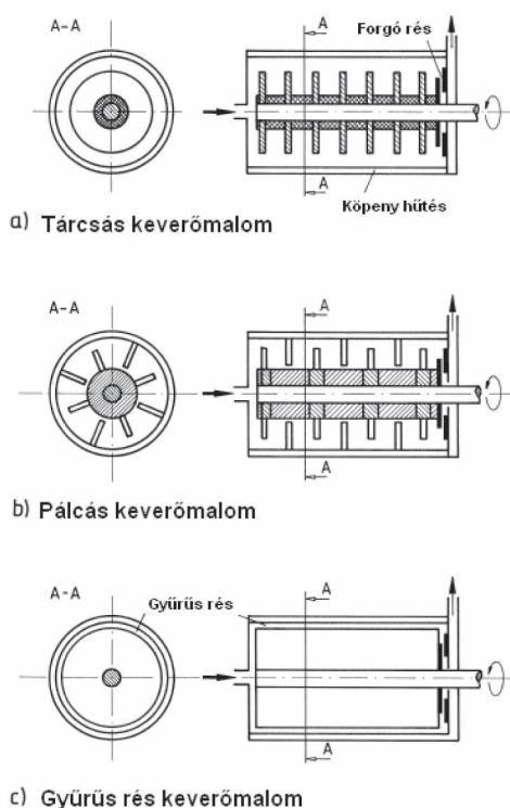
1. ábra Folyamatos üzemű nedves keverőmalom típusok [3] Fig 1. Different types of continuous operation wet stirred ball mill
