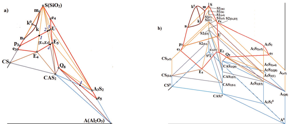
Fig. 2. XY projection (a) and 3D model (b) of fragment of system S-A-C phase diagram 2. ábra Az S-A-C fázisdiagram egy töredékének XY vetülete (a) és 3D modellje (b)
