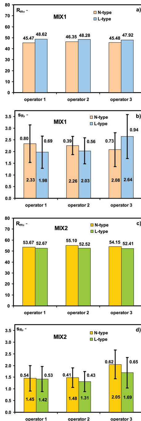
Fig. 6. Repeatability and reproducibility analysis of the rebound hammer test 6. ábra Ismételhetőségi és reprodukálhatósági jellemzők Schmidt kalapácsos vizsgálátra vonatkozóan
