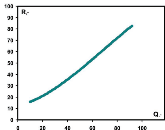
Fig. 3. Relationship between rebound index R and rebound index Q [7] 3. ábra Az R és a Q visszapattanási érték kapcsolata [7]
