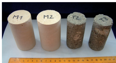
Fig. 1. Cylindrical coarse limestone and rhyolite tuff specimens 1. ábra Hengeres durva mészkő és riolitufa próbatestek
