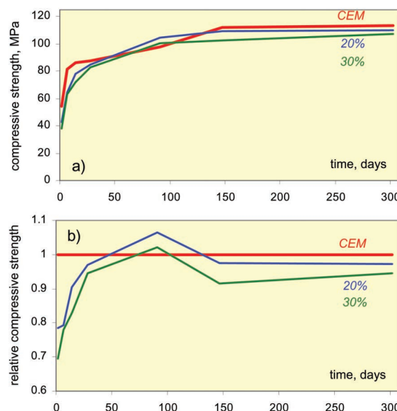
Fig. 7. Compressive strength and relative compressive strength of specimens with green WGP 7. ábra Nyomószilárdság és relatív nyomószilárdság fejlődése a zöld színű hulladék üveg por kiegészítővel
