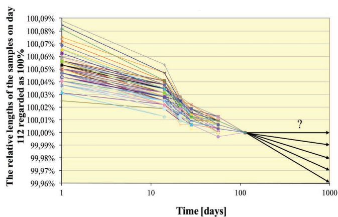
Fig. 16. The deformation process of samples made with CEM I 32.5 N over a logarithmic timescale, with the dimensions of the prisms on day 112 regarded as 100%. The arrows indicate the possible values for deformation projected to day 1000, by continuing the trends. The question mark is there because all projections of this nature need to be validated through real measurements 16. ábra A CEM I 32,5 N cementből készült hasábok alakváltozási folyamata logaritmikus időskálán szemlélítve, ha a hasábok 112 napos méreteit tekintjük 100%-nak. A nyilakkal az eddigi trend folytatódása esetén az 1000 napos korra prognosztizálható alakváltozás lehetséges értékeit jelöljük. A „?” utalás arra, hogy minden prognózist csak valós mérési eredmények hitelesíthetnek
