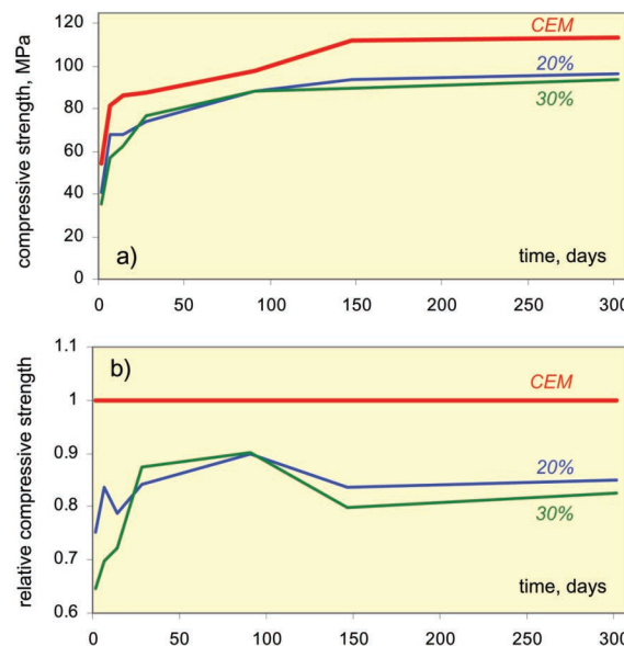
Fig. 6. Compressive strength and relative compressive strength of specimens with flint WGP 6. ábra Nyomószilárdság és relatív nyomószilárdság fejlődése a fehér színű hulladék üveg por kiegészítővel
