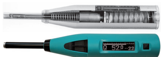
Fig. 1. Original Schmidt rebound hammer and Silver Schmidt rebound hammer 1. ábra Az eredeti Schmidt kalapács és a Silver Schmidt kalapács
