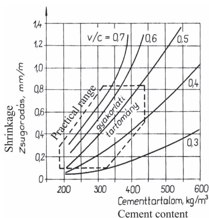
Fig. 17. Depiction of shrinkage with influencing parameters [7] 17. ábra A zsugorodást befolyásoló egyes tényezők hatása [7]
