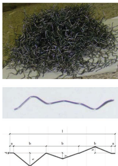
Fig. 5. 3D deformed, twisted steel fibre, PetiX S60 5. ábra Három dimenzióban megmunkált PetiX S60 acélszál
