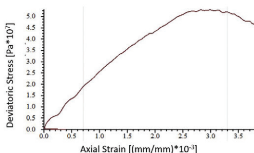
Fig. 5. The deviatoric stress vs. the axial strain during the compression test procedure 5. ábra A deviátoros feszültség és a tengelyirányú fajlagos összenyomódás kapcsolata
