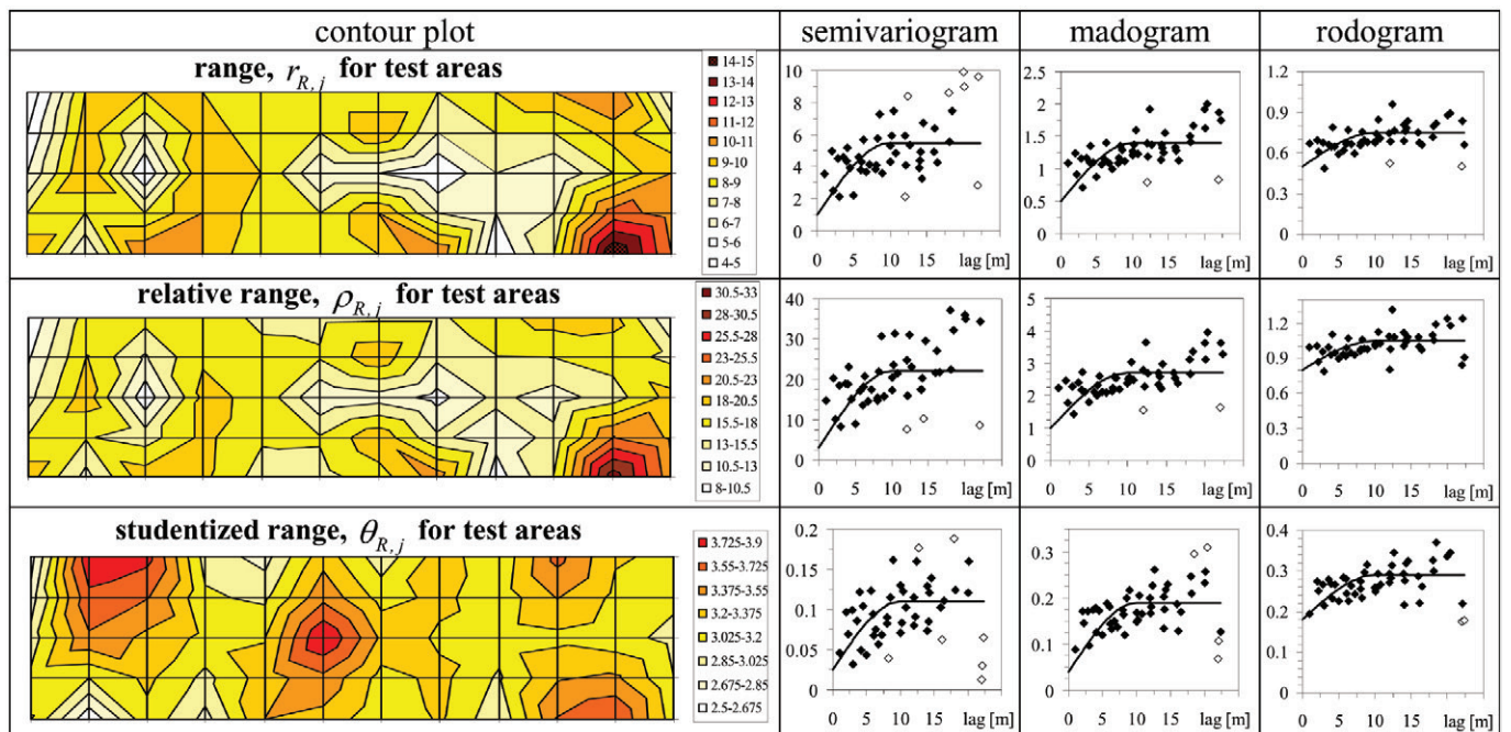
Fig. 4. Variographic analysis for the statistical dispersion parameters 4. ábra Terjedelem paraméterek variográfiái vizsgálata
