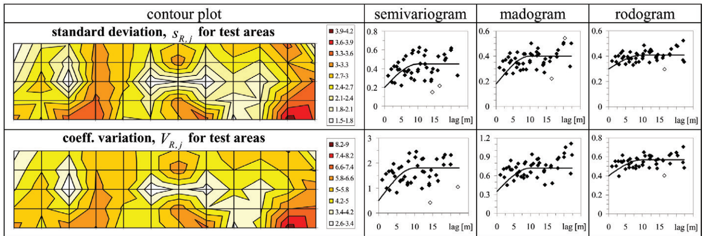
Fig. 3. Variographic analysis for the statistical variance parameters 3. ábra Variancia paraméterek variográfiái vizsgálata
