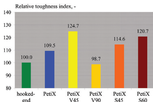
Fig. 7. Relative toughness indices of SFRC specimens 7. ábra SFRC hasákok relatív szívóssági indexei
