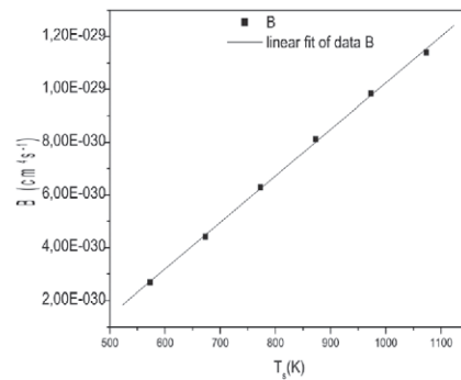
Fig. 4. Variation of the coalescence parameter (B)
