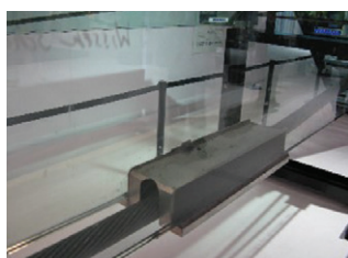
12. ábra 9 m-es feszítávú járható feszített üvegszerkezet. Fig. 12. Prestressed glass bridge with 9 m span.
