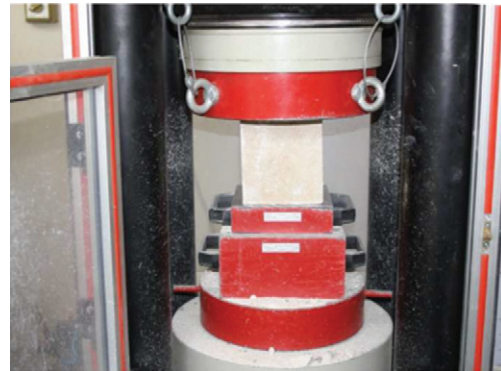
Fig. 4. Compressive strength testing 4. ábra Nyomószilárdság vizsgálata
