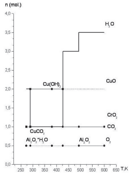
Fig. 2. Influence of temperature on phase-chemical transformations in Al-Cu-Cr-O catalysis system 2. ábra A hőmérséklet hatása a fázis-kémiai átalakulásokra Al-Cu-Cr-O katalízis rendszerben
