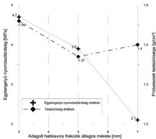
7. ábra Geopolimer kompozit próbatestek 7 napos nyomószilárdságának és testsűrűségének változása a habkavics méretfrakciók átlagos méretének függvényében
