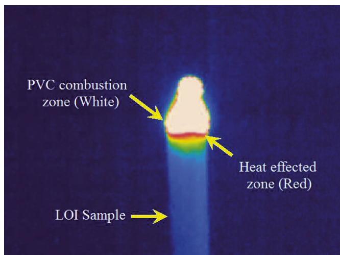
Fig. 2. FLIR thermal gradient image for heat affected zone (HAZ) in plasticised PVC L. O. I. test 2. ábra A hőhatásnak kitett zóna (HAZ) FLIR termikus gradiens képe a lágyított PVC L. O. I. vizsgálatá közben
