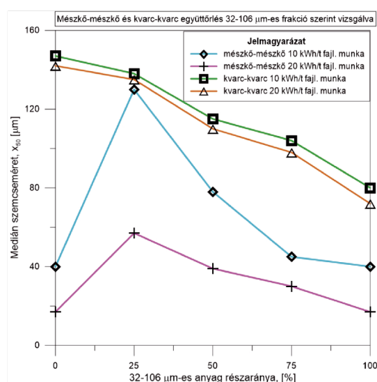
13. ábra Medián szemcseméret változása a 32-106 \mu\text{m} -es frakció részaránya szerint kvarc és mészkő különböző méretű frakcióinak együttőrlésekor
