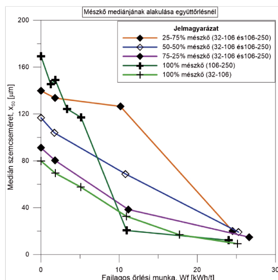
12. ábra Medián változása különböző méretű mészkő frakciók együttőrlésekor
