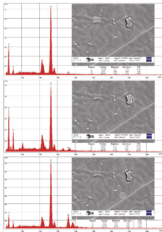
Fig. 6. SEM - energy dispersive X-ray microanalysis for HAZ in burned plasticised PVC + 3% \text{Sb}_2\text{O}_3 LOI sample 6. ábra SEM - energia diszperzív röntgen mikroanalízis a HAZ az elégett lágyított PVC-ben. \text{Sb}_2\text{O}_3 tartalom 3%
