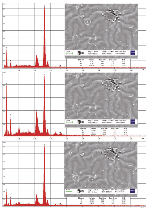
Fig. 5. SEM - energy dispersive X-ray microanalysis for HAZ in burned plasticised PVC + 1% \text{Sb}_2\text{O}_3 LOI sample 5. ábra SEM - energia diszperzív röntgen mikroanalízis a HAZ az elégett lágyított PVC-ben. \text{Sb}_2\text{O}_3 tartalom 1%
