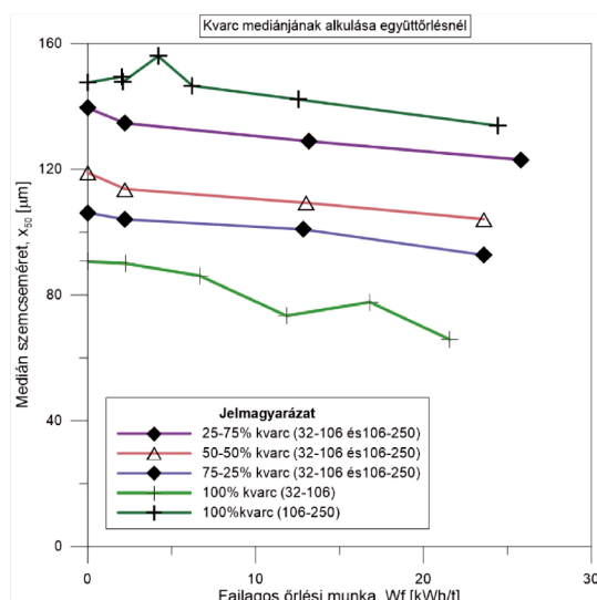
11. ábra Az őrlmény mediánjának alakulása különböző szemcseméretű kvarc frakciók együttőrlésénél
