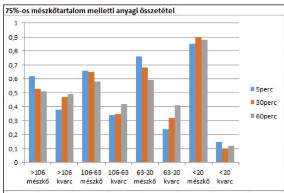
10. ábra Az őrlmény anyagi összetétele kvarc-mészko együttörlés esetén Fig. 10 Material composition of the ground material in case of quartz-limestone intergrinding
