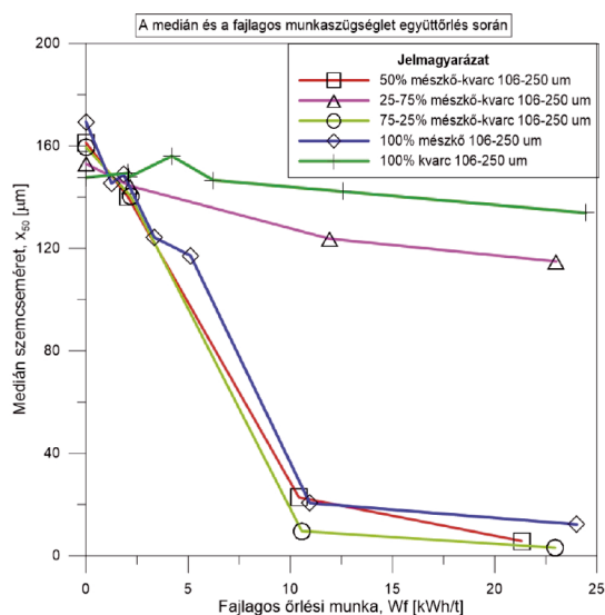
7. ábra A medián változása a fajlagos őrlési munkaszükséglet függvényében mészkő-kvarc együttőrleése során Fig. 7 The median particle size as a function of the specific grinding work in case of limestone-quartz intergrinding
