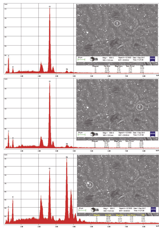
Fig. 7. SEM - energy dispersive X-ray microanalysis for HAZ in burned plasticised PVC + 5% \text{Sb}_2\text{O}_3 LOI sample 7. ábra SEM - energia diszperzív röntgen mikroanalízis a HAZ az elégett lágyított PVC-ben. \text{Sb}_2\text{O}_3 tartalom 5%
