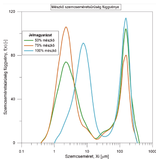
8. ábra 106-250 \mu\text{m} -es frakció szemcseméret-sűrűségfüggvénye 60 perces mészkő-kvarc együttőrleésnél Fig. 8 Particle size density function of 106-250 \mu\text{m} fraction at 60 min limestone-quartz intergrinding
