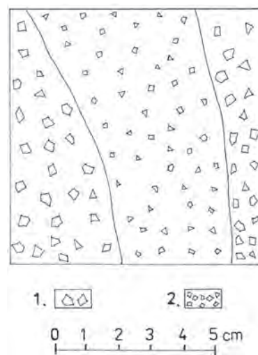
6. ábra A durva és finomabb szemcsés bázikus magmás kőzet kontaktusa 1- gabbró 2- finomabb szemcsésű diabáz típusú vulkanit
